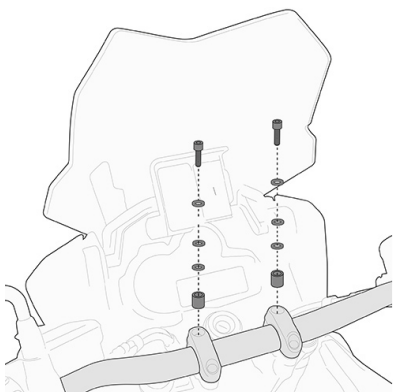
03SKITK Spezifisches Kit für die Montage der Smart Bar KS900A
